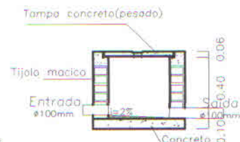
CORTE AA'
