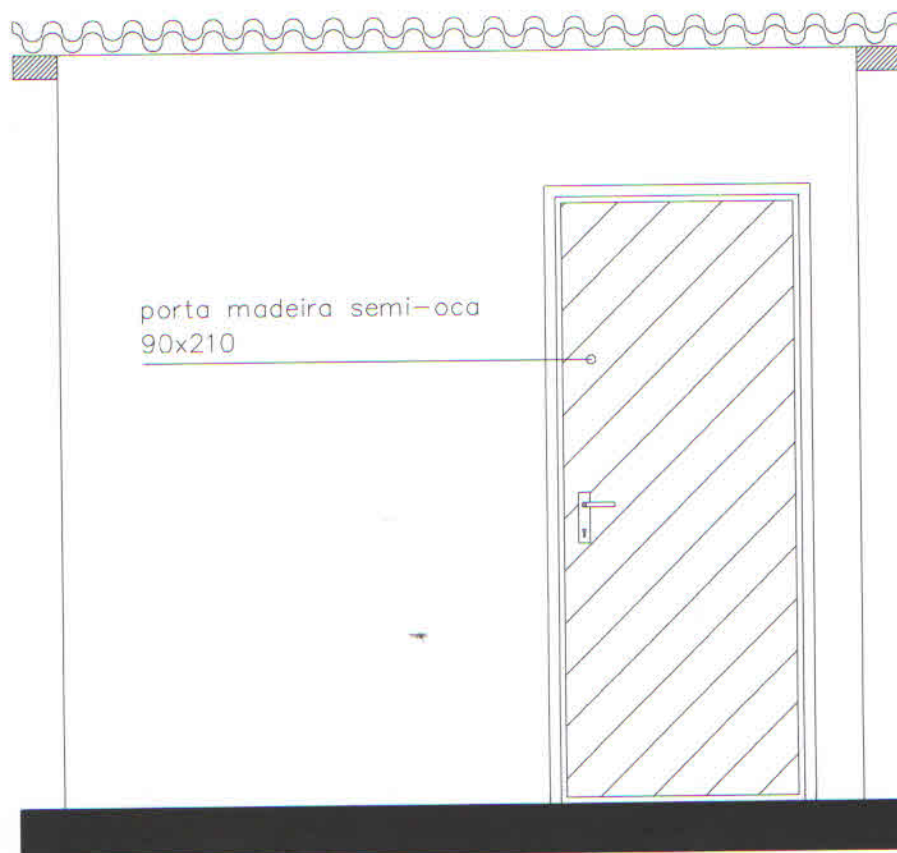
FACHADA FRONTAL
