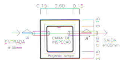
PLANTA BAIXA
