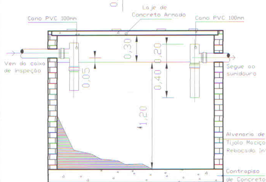
CORTE AA' FOSSA SÉPTICA
